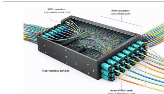
圖 5：新富生光電 XFS 光纖配線產品圖
