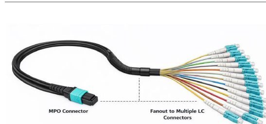
圖 4：新富生光電 XFS MPO Connector
