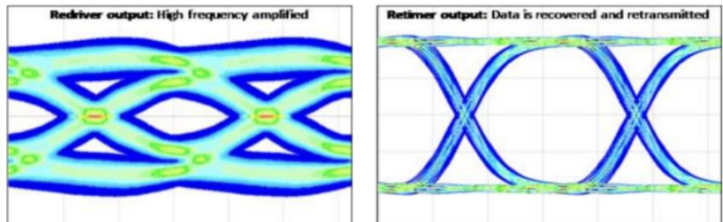
圖 10：Redriver (左)單純將線路內訊號一併放大，Retimer (右)對訊號進行調節並放大
